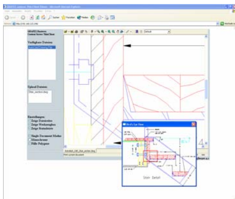
AutoCAD Datei zoomen mit Bird's Eye View
