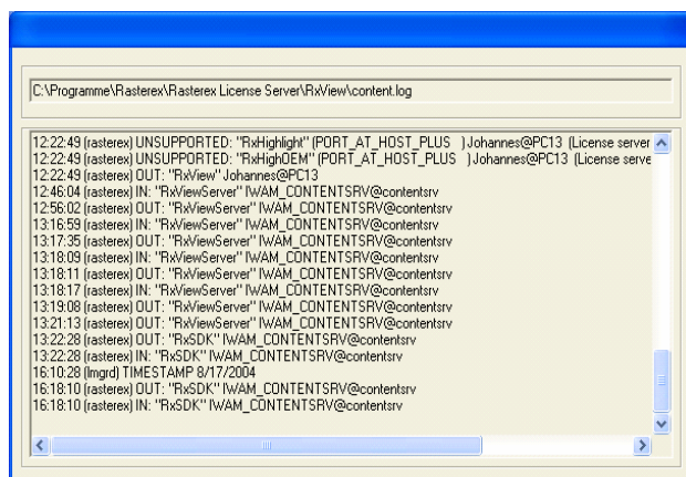
Lizenzverwaltung über Flex LM
